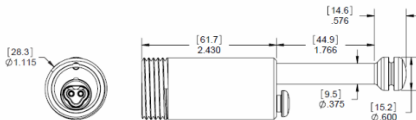
Размеры с колпачком
