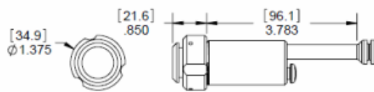
Размеры с колпачком
